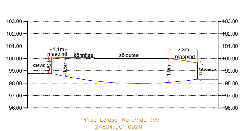
Lõige nr.3 Ristumine riigiteega nr 14135 Laiuse-Kuremaa tee km 1.54
