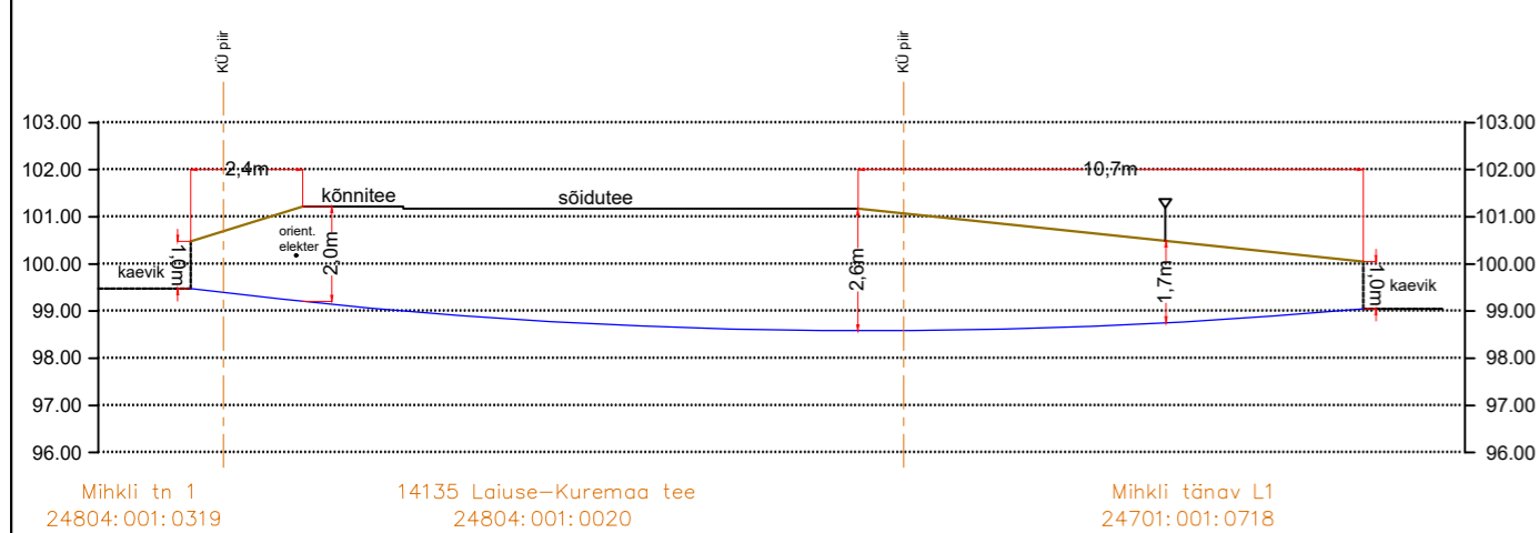
Lõige nr.4 Ristumine riigiteega nr 14135 Laiuse-Kuremaa tee km 1.46
