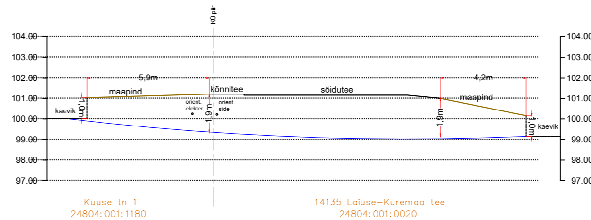
Lõige nr.7 Ristumine riigiteega nr 14135 Laiuse-Kuremaa tee km 1.22
