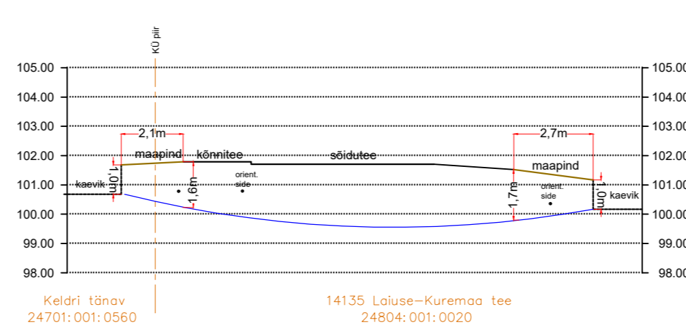
Lõige nr.5 Ristumine riigiteega nr 14135 Laiuse-Kuremaa tee km 1.37
