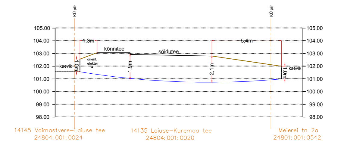
Lõige nr.11 Ristumine riigiteega nr 14135 Laiuse-Kuremaa tee km 0.76
