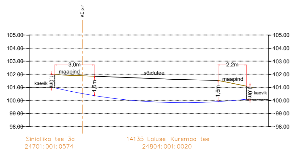
Lõige nr.1 Ristumine riigiteega nr 14135 Laiuse-Kuremaa tee km 2.04
