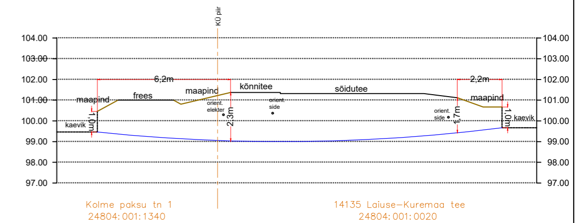
Lõige nr.9 Ristumine riigiteega nr 14135 Laiuse-Kuremaa tee km 0.99
