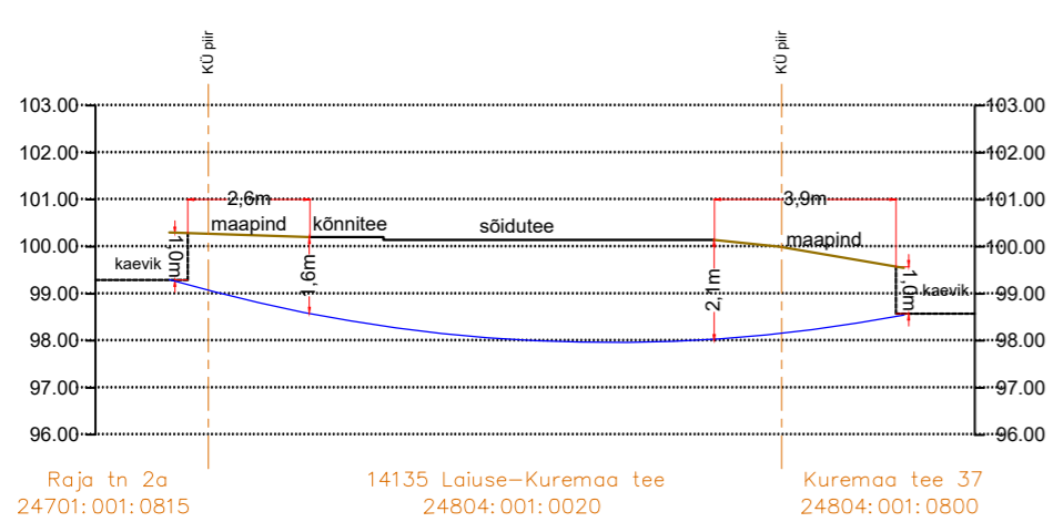
Lõige nr.3 Ristumine riigiteega nr 14135 Laiuse-Kuremaa tee km 1.54
