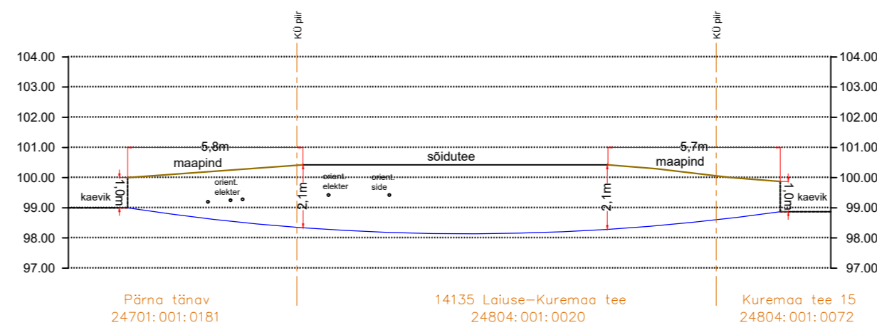
Lõige nr.8 Ristumine riigiteega nr 14135 Laiuse-Kuremaa tee km 1.09
