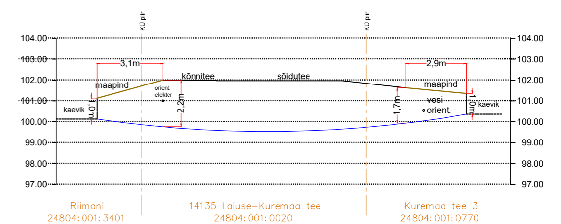
Lõige nr.10 Ristumine riigiteega nr 14135 Laiuse-Kuremaa tee km 0.82
