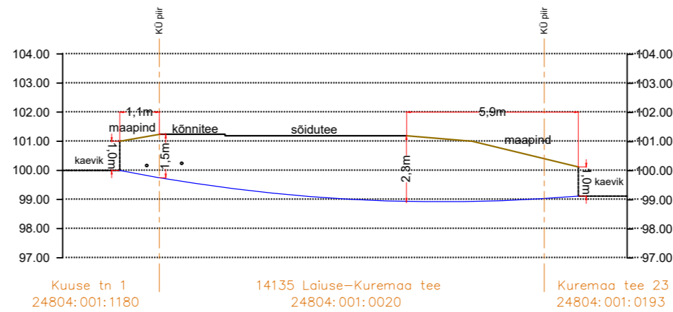
Lõige nr.6 Ristumine riigiteega nr 14135 Laiuse-Kuremaa tee km 1.28
